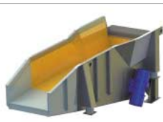
Schwingförderer mit Unwuchtantrieb Vibrating trough conveyor with unbalanced motor
